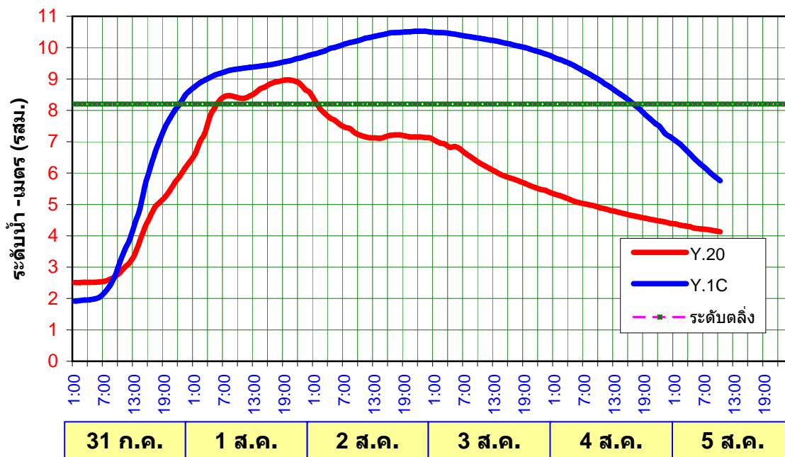
ระดับน้ำมรายชั่วโมงที่สถานีY.20และสถานีY.1C วันที่ 31- 5 ส.ค. 2554
