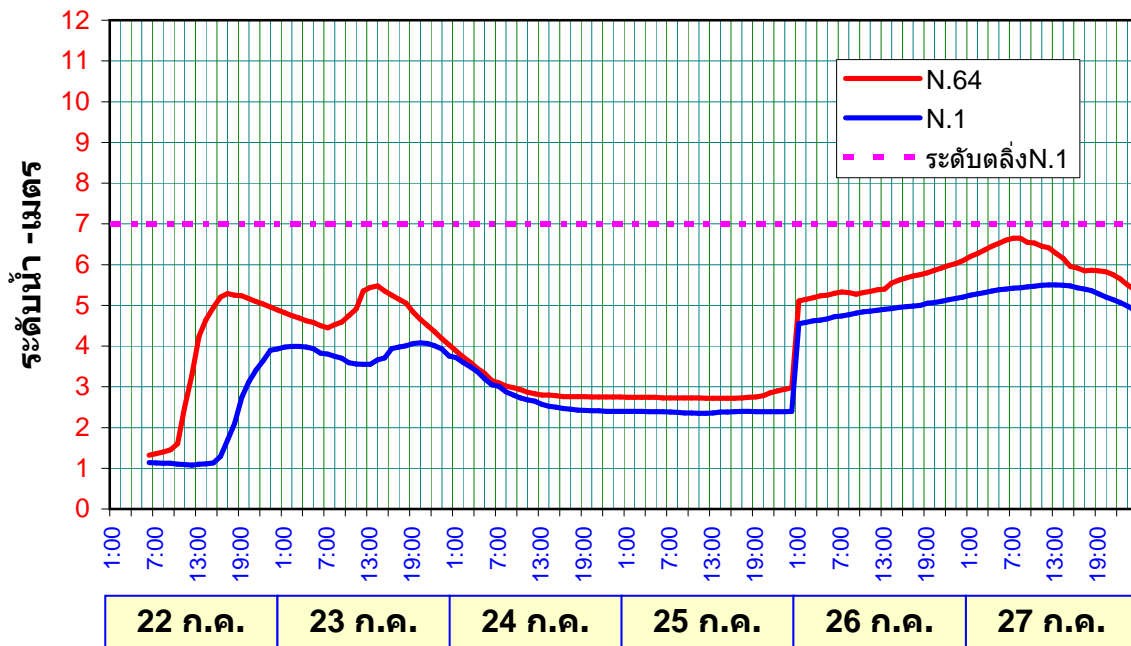
ระดับน้ำน่านรายชั่วโมงที่สถานีN.64และสถานีN.1 วันที่ 22 - 27 ก.ค. 2553
