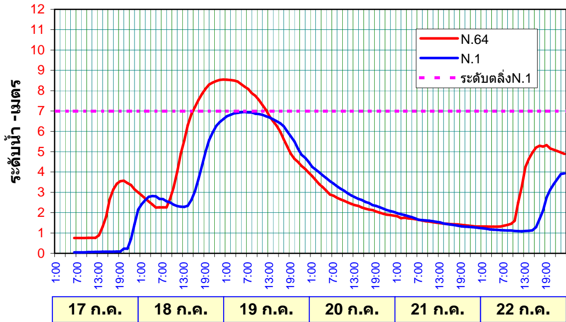
ระดับน้ำน่านรายชั่วโมงที่สถานีN.64และสถานีN.1 วันที่ 17 - 22 ก.ค. 2553
