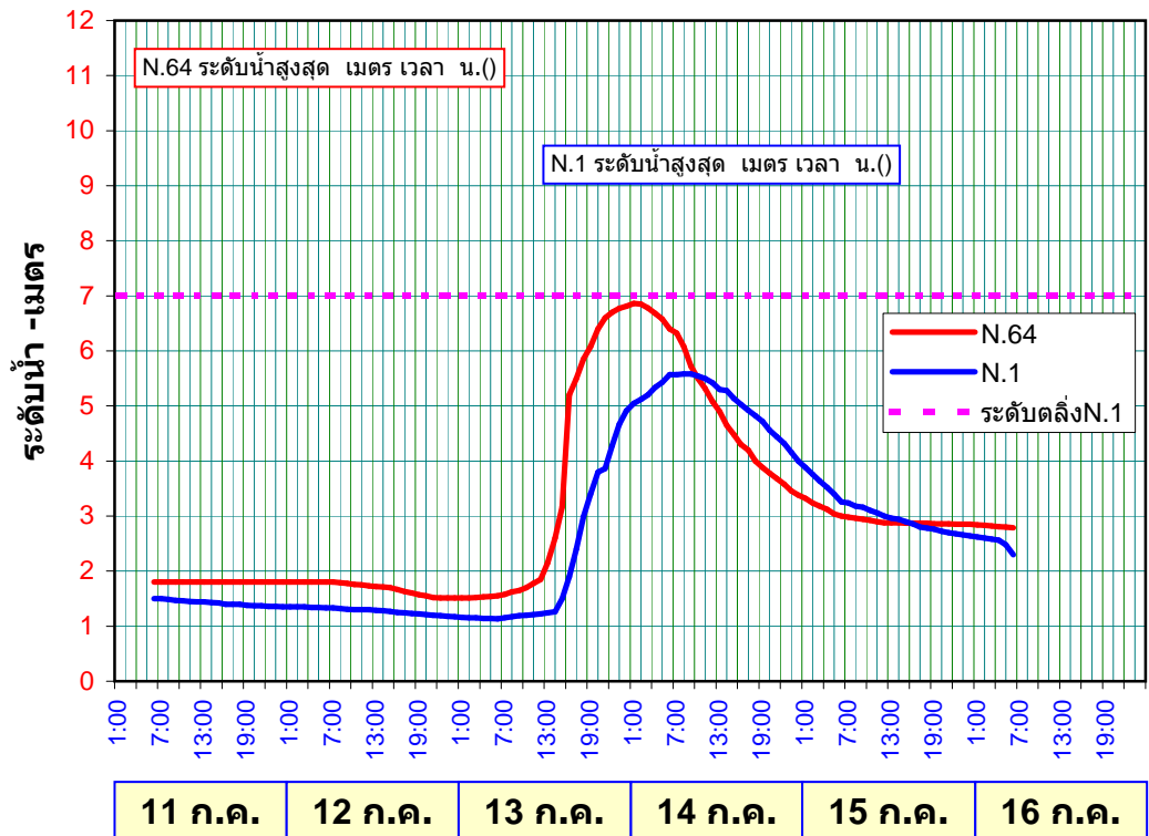
ระดับน้ำน่านรายชั่วโมงที่สถานีN.64และสถานีN.1 วันที่ 11-16 ก.ค. 2552
