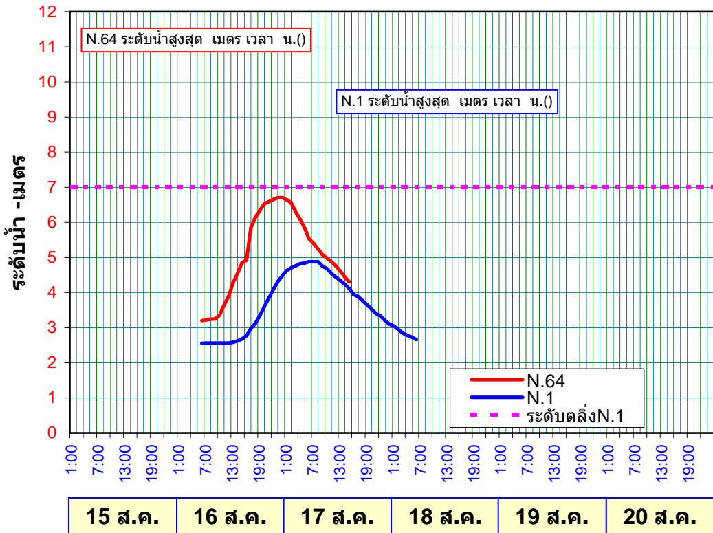
ระดับน้ำน่านรายชั่วโมงที่สถานีN.64และสถานีN.1 วันที่ 15-20 ส.ค. 2552
