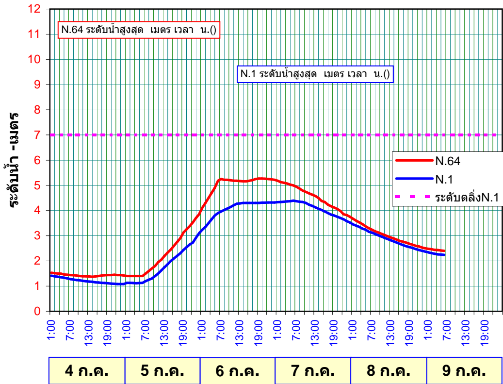
ระดับน้ำน่านรายชั่วโมงที่สถานีN.64และสถานีN.1 วันที่ 04-09 ก.ค. 2552
