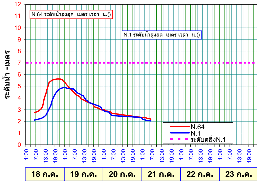
ระดับน้ำน่านรายชั่วโมงที่สถานีN.64และสถานีN.1 วันที่ 18-23 ก.ค. 2552
