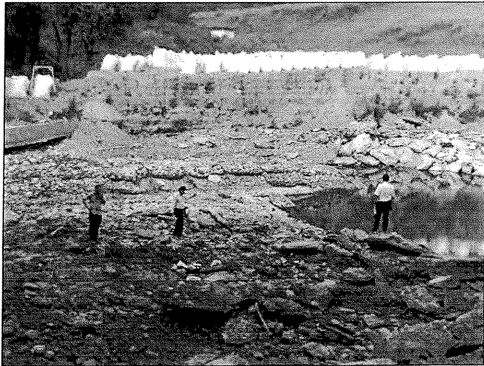
อาคารทางระบายน้ำสันอ่างเก็บน้ำน้ำพอง อำเภอสันติสุข จังหวัดน่าน ที่ถูกน้ำกัดเซาะบริเวณด้านท้ายน้ำพังเสียหาย
