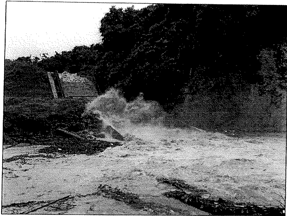
อาคารทางระบายน้ำล้นอ่างเก็บน้ำน้ำพอง อำเภอสันติสุข จังหวัดน่าน ที่ถูกน้ำกัดเซาะบริเวณคันท้ายน้ำพังเสียหาย
